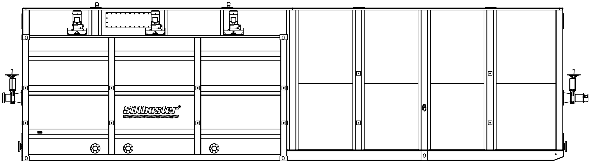
MT30 L: 6057mm W: 2438mm H: 3121mm H: 2886mm (BRIM) MT100 L: 12342mm W: 3189mm H: 3506mm
