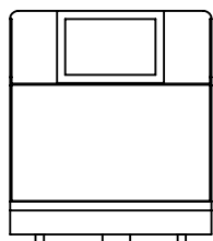
DOSING SKID L: 600mm W: 1220mm H: 1400mm
